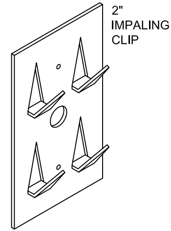
2 IMPALING CLIPS CX-01 SCALE: NA
