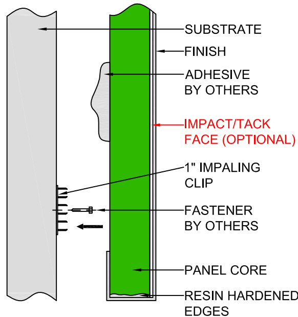
2 IMPALING CLIPS CX-01 SCALE: NA
